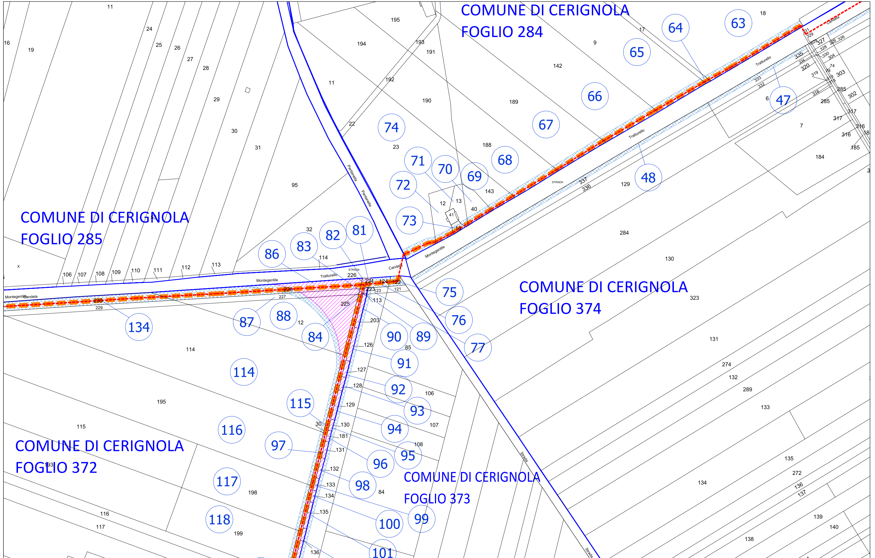
TAV. 4 - scala 1:2000
