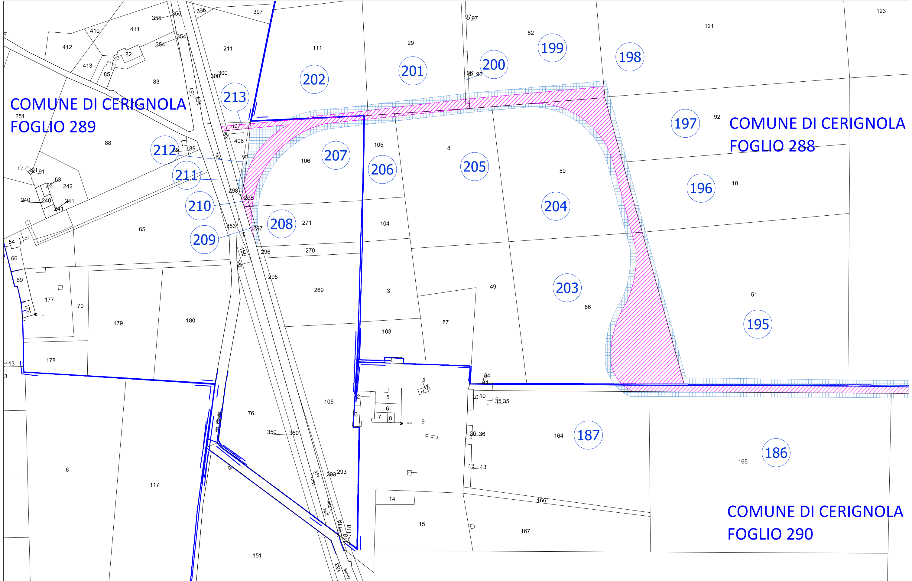
TAV. 9 - scala 1:2000
