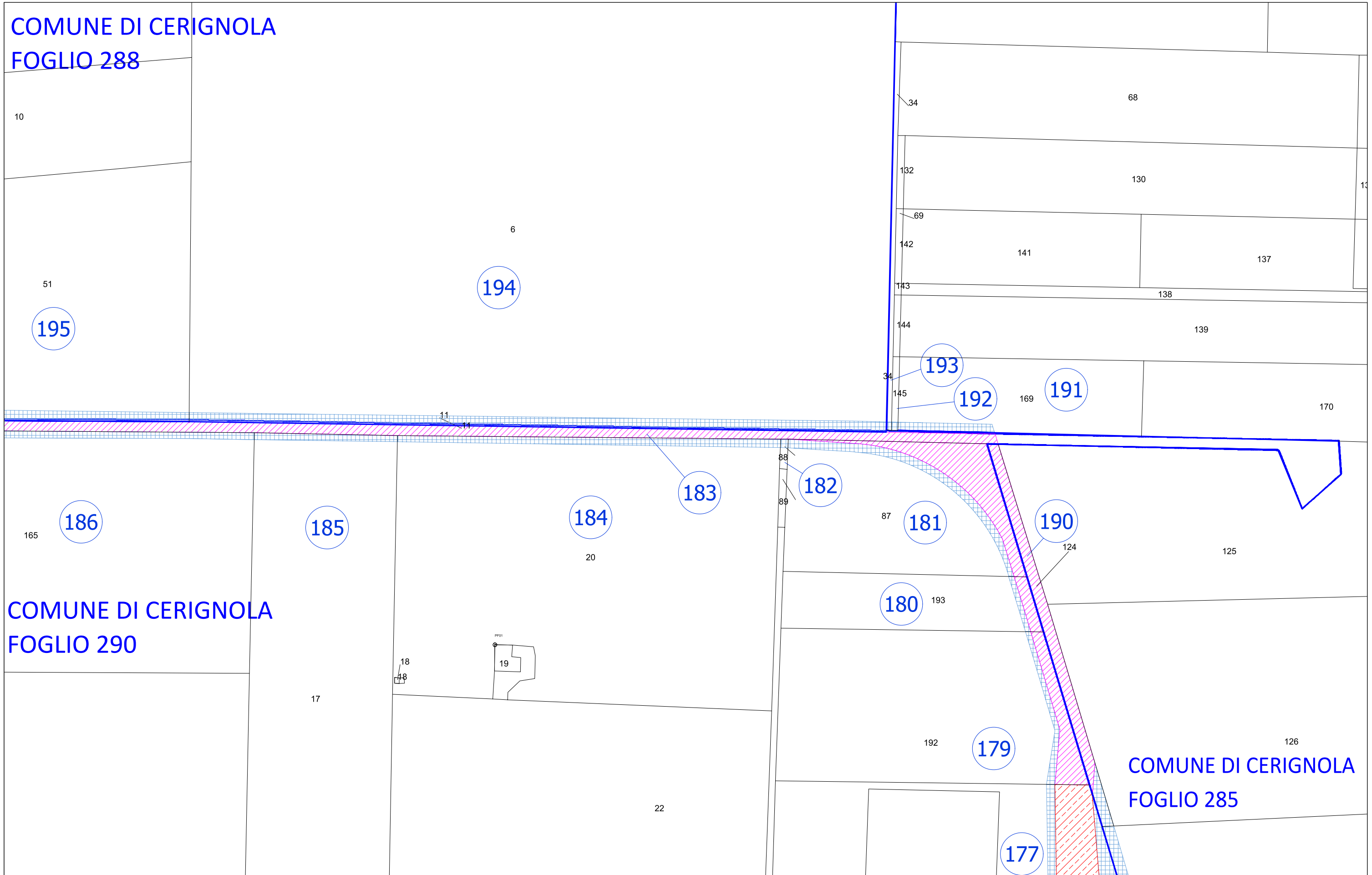
TAV. 8 - scala 1:2000
