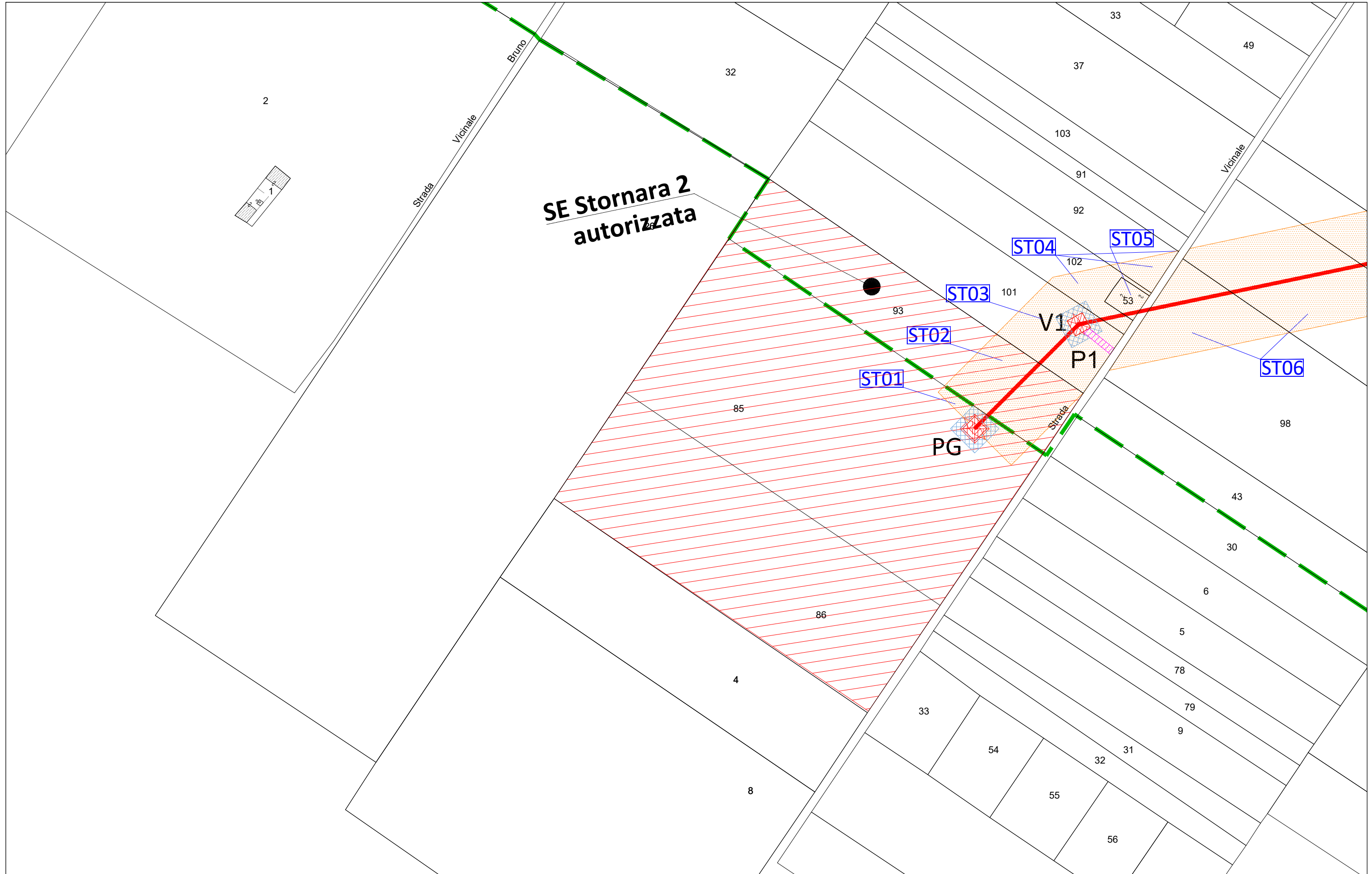
TAV. 49 - scala 1:2000
