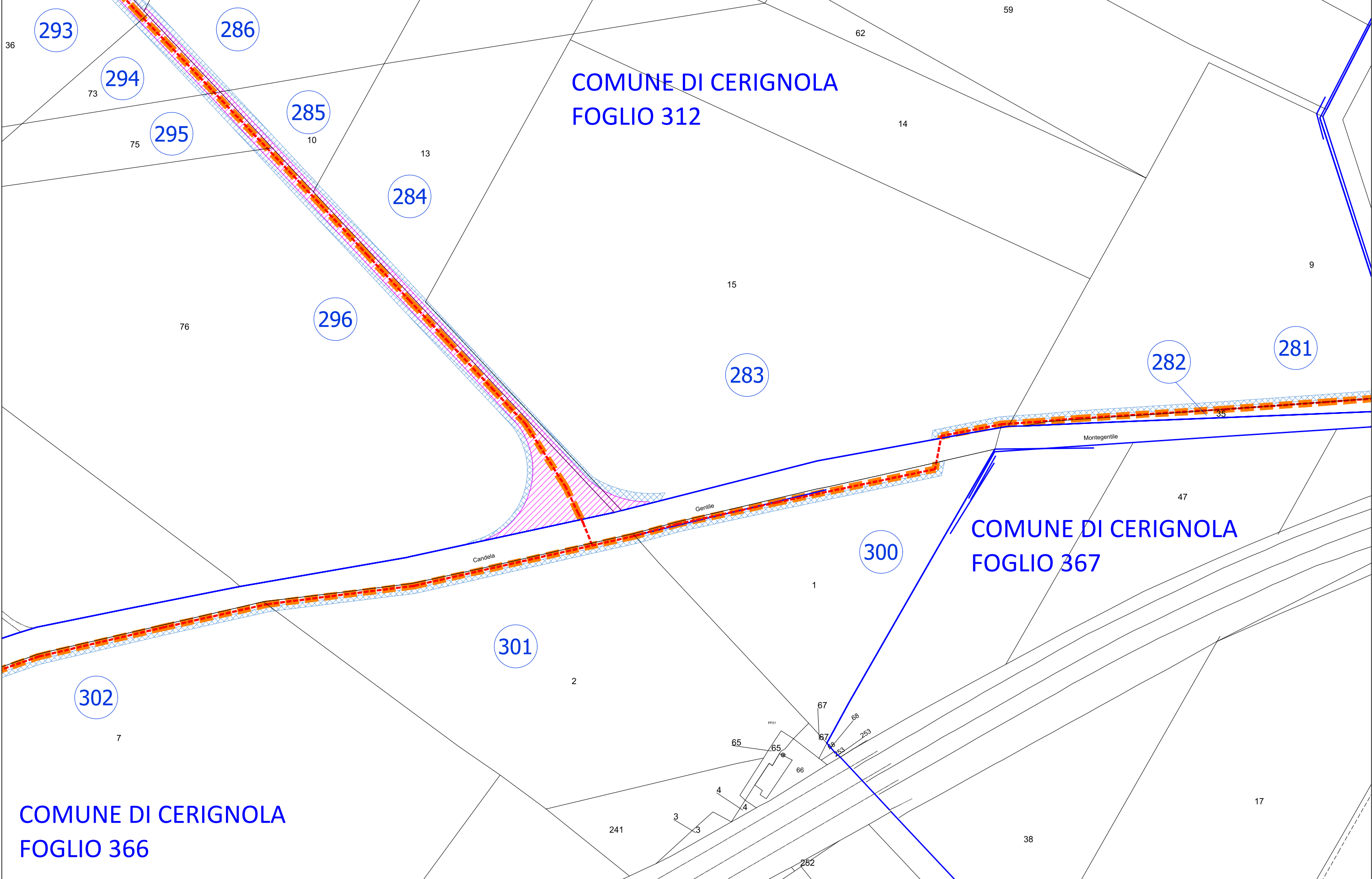
TAV. 20 - scala 1:2000
