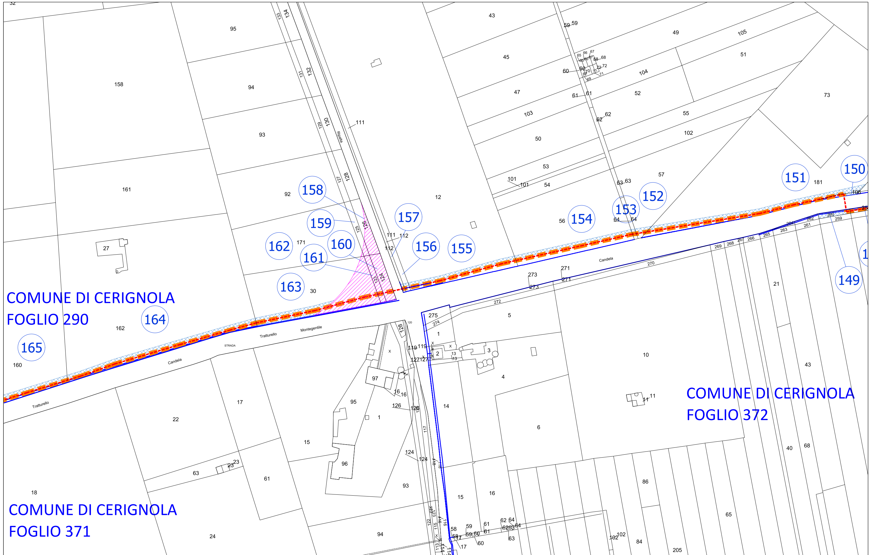
TAV. 10 - scala 1:2000
