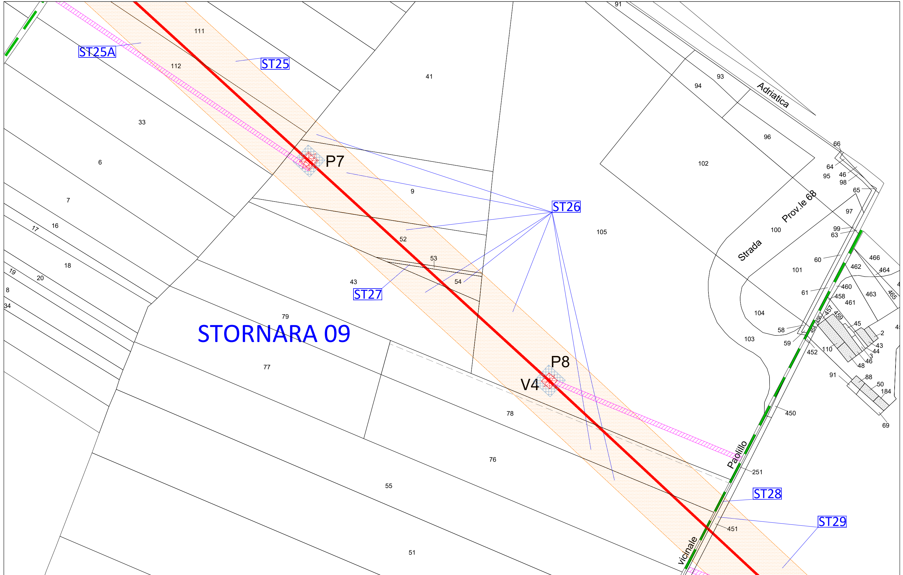
TAV. 45 - scala 1:2000
