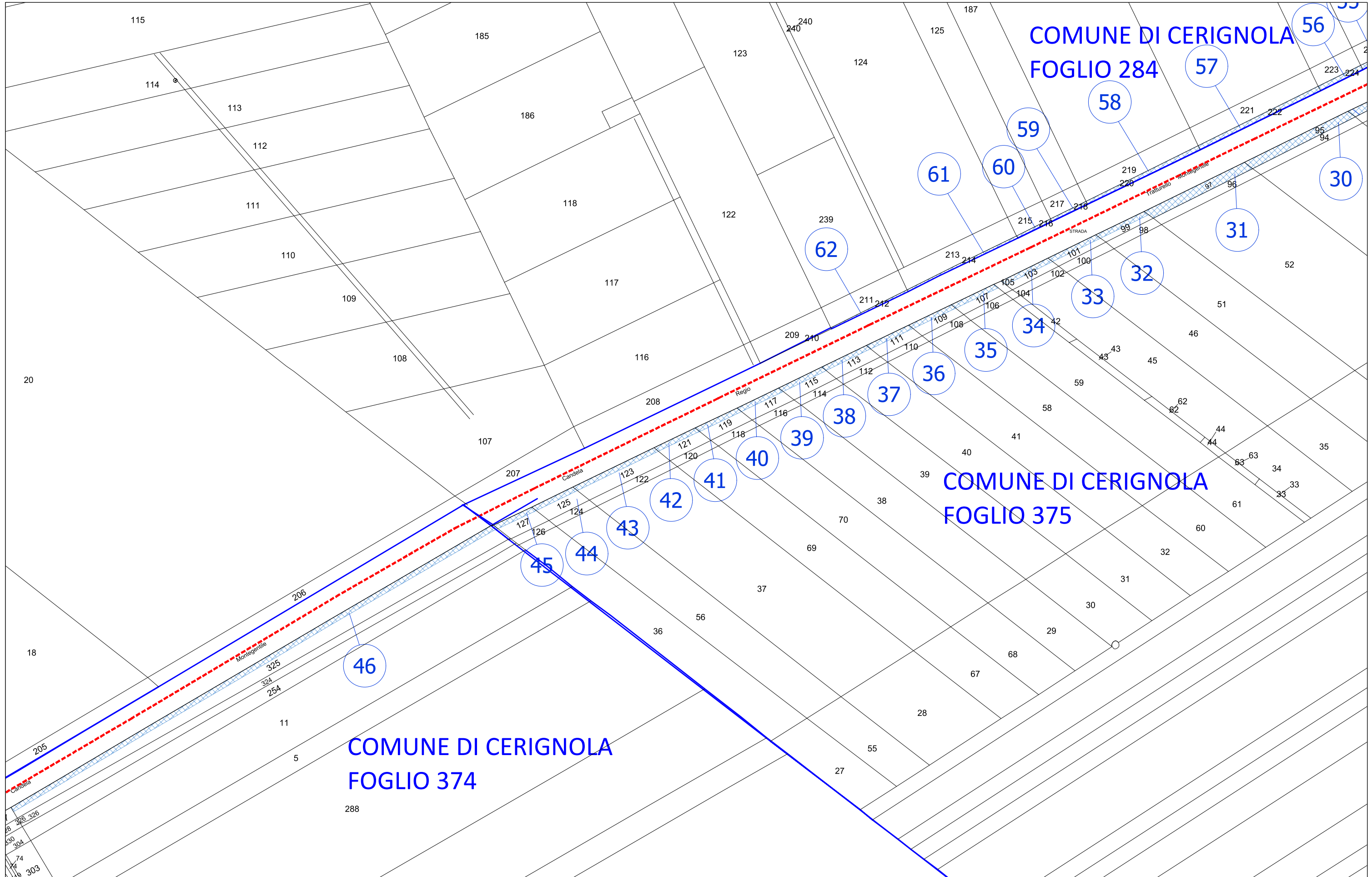
TAV. 3 - scala 1:2000
