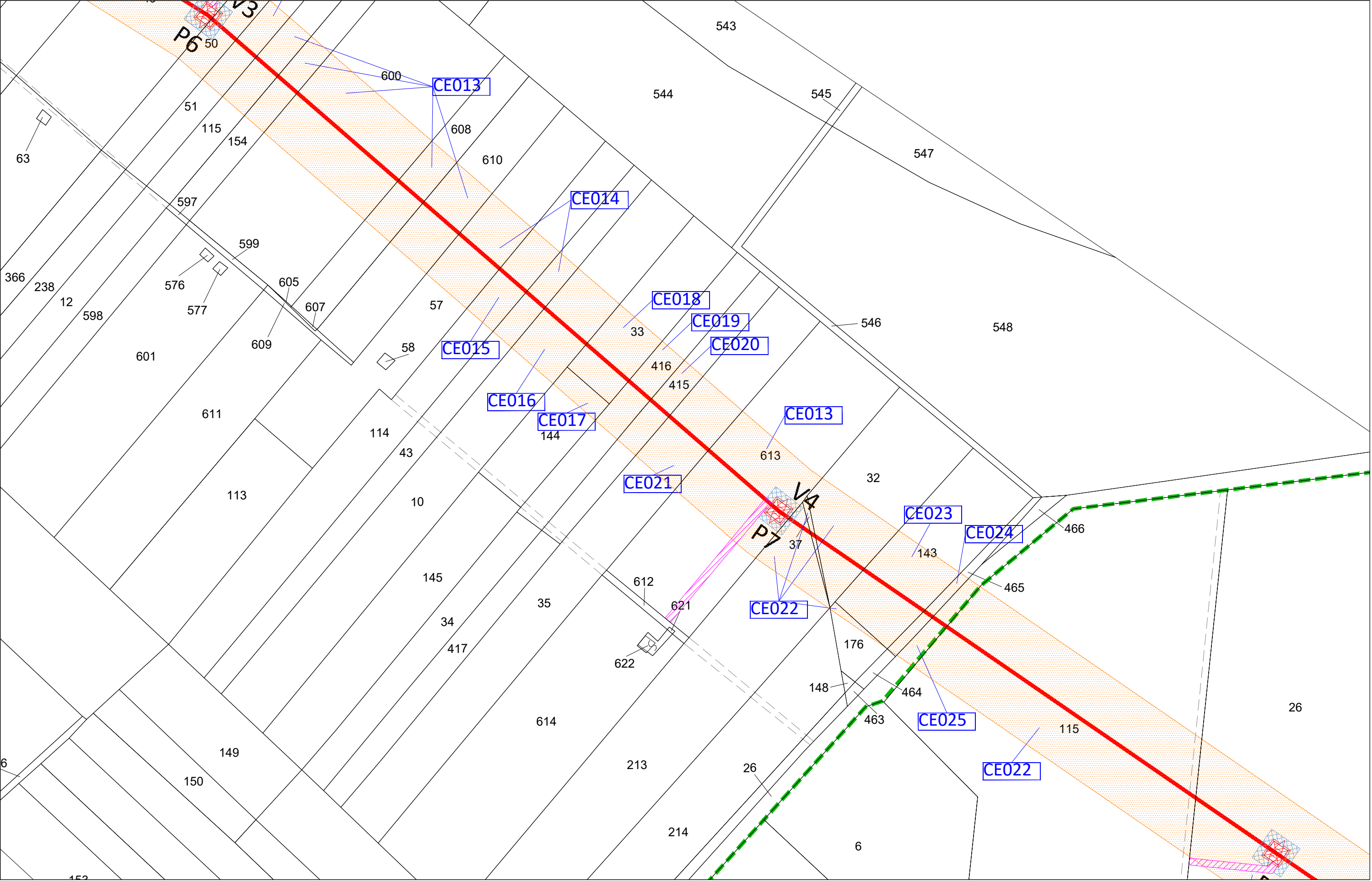
TAV. 38 - scala 1:2000
